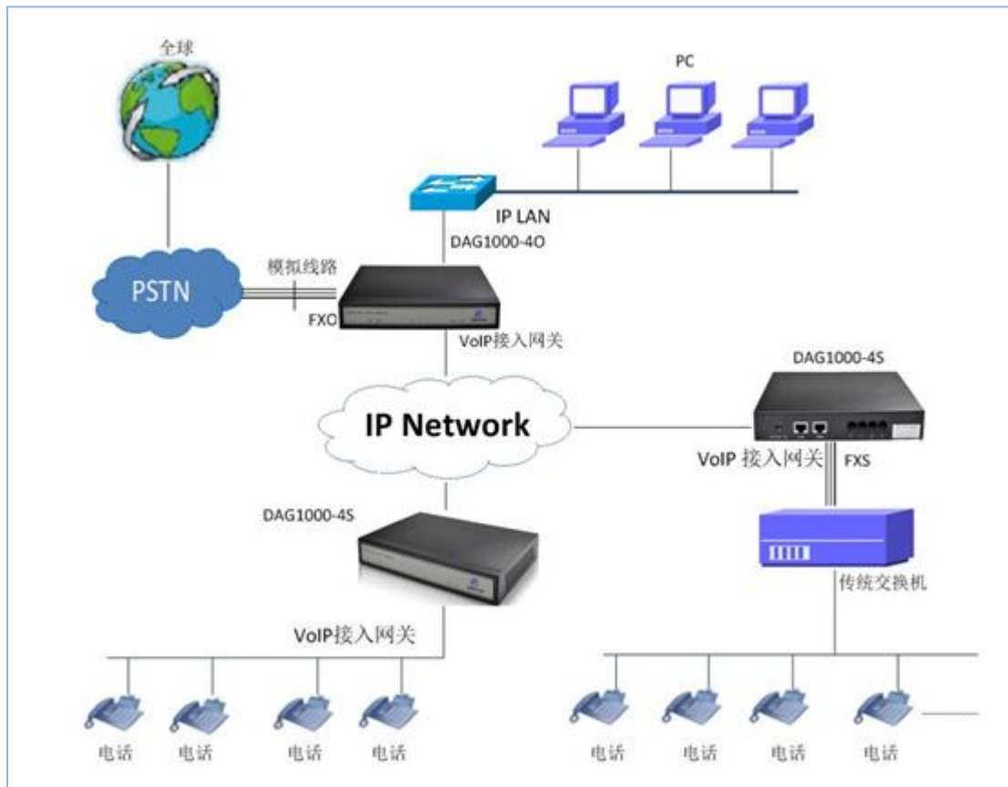
图 1-3: 应用图
