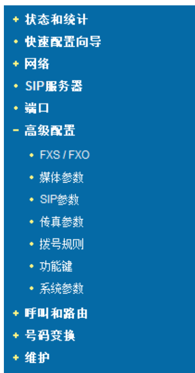
图 4-2-1: 导航树
