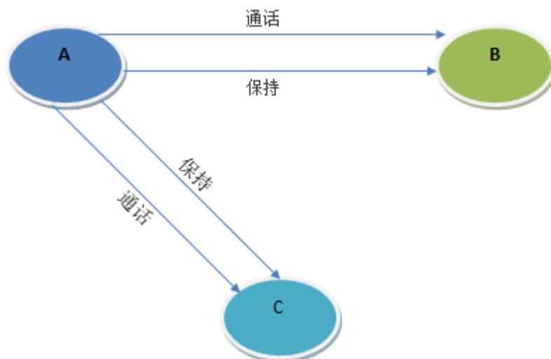
图 2-1：三方通话
