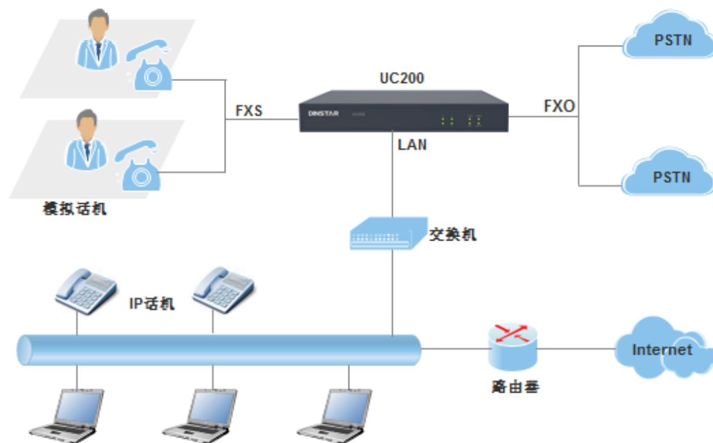
图 1-1 UC200-2S20 应用场景
