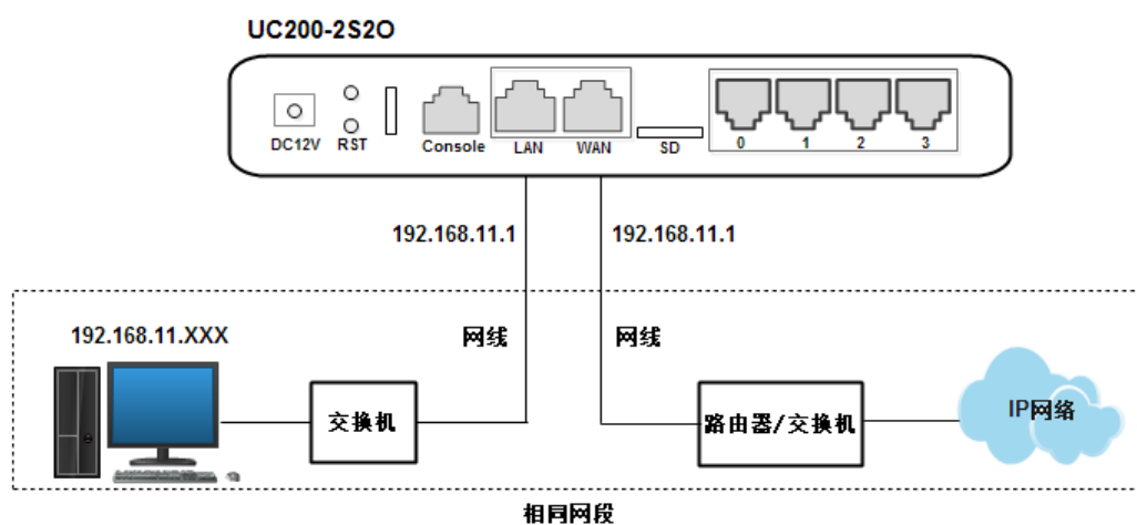
图 2-2 桥接模式下的网络连接图
