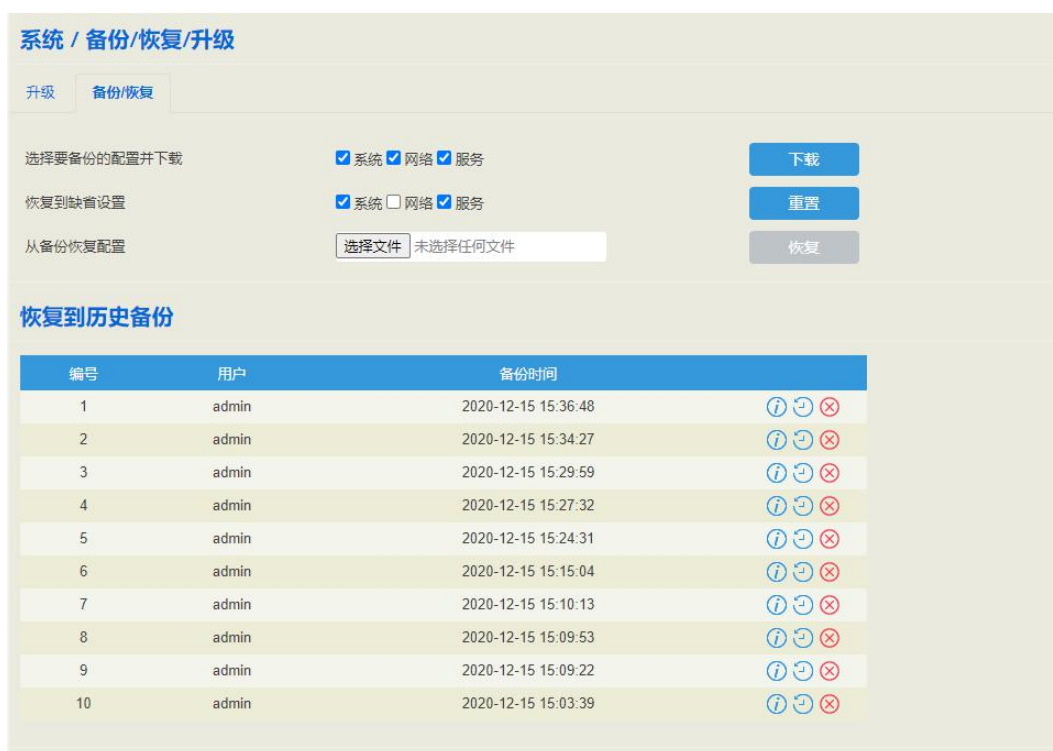
图 5-3-8 备份/恢复
